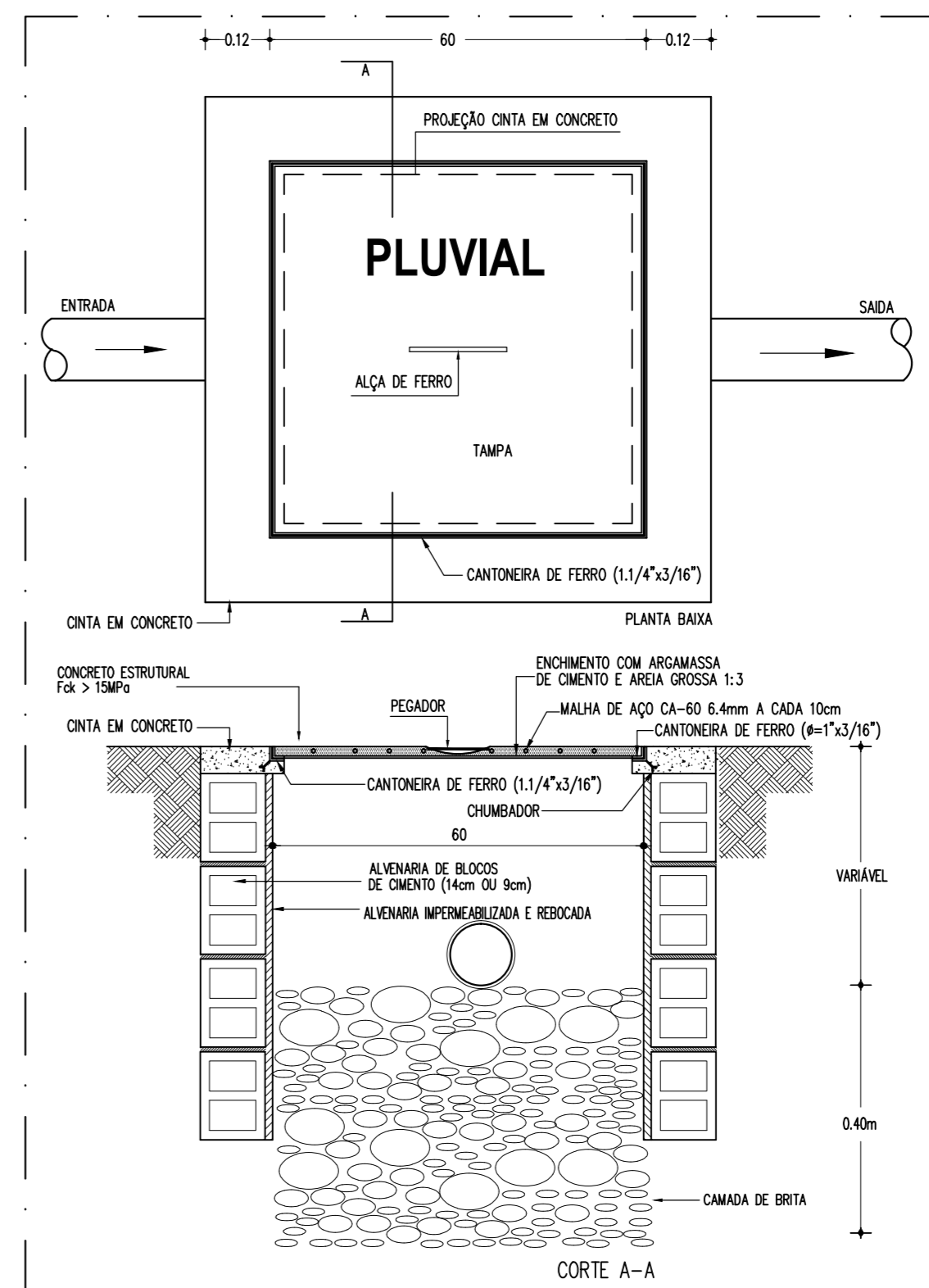
03 DETALHE DA CAIXA DE AREIA ESC. SEM
