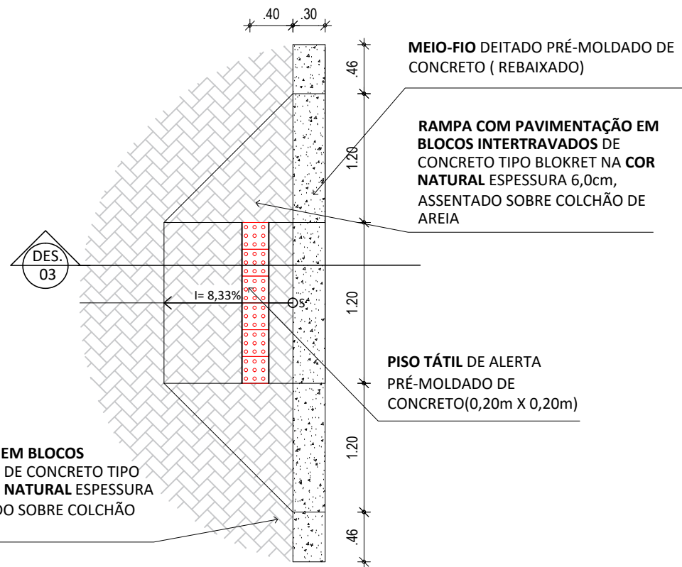
3 PLANTA BAIXA RAMPA ESC.: 1:50
