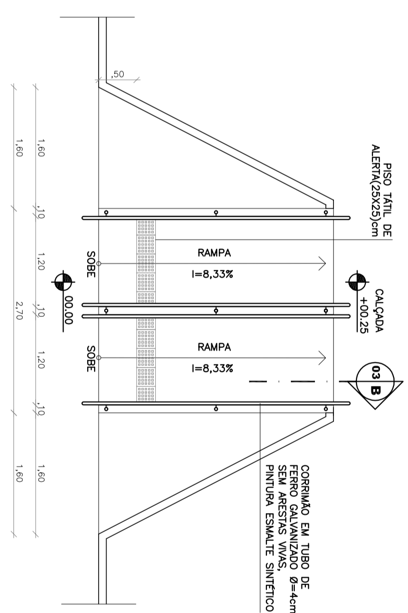
02 RAMPA PNE TIPO 2 - PLANTA ESCALA: 1:50
